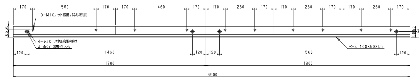
基礎図
